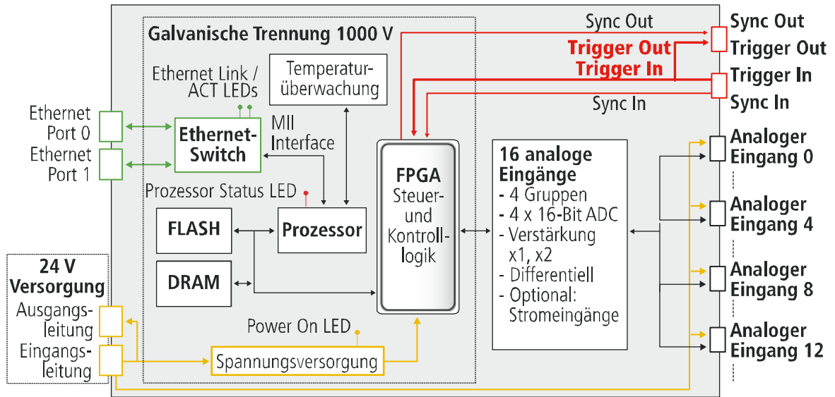
Abb. 2-1: MSX-E3011: Blockschaltbild
