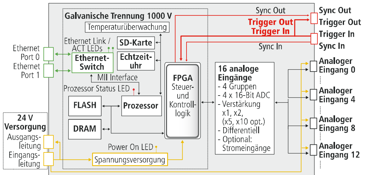
Abb. 2-2: MSX-E3021: Blockschaltbild
